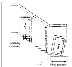
6. schodisko stáčajúce sa pod uhlom 180° s podestou
