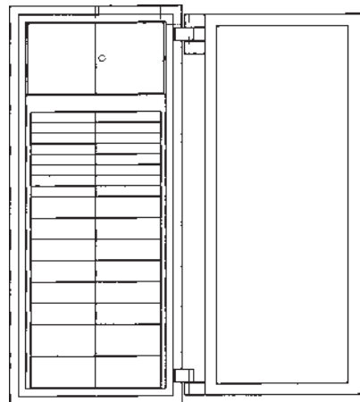
Wertschutzschrank Modellreihe 1901 mit 32 Mietfächern (2 x LSN 0016) und versperbarem Innenfach
